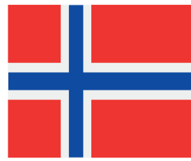
Norwegia
